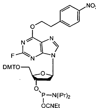
2-F-dI-CE Phosphoramidite
